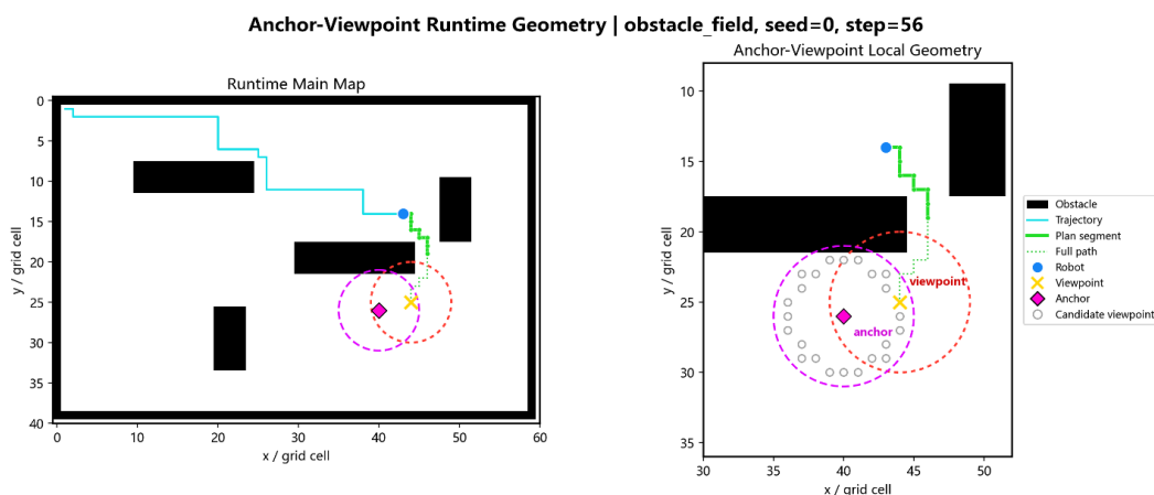
图 3-1 Anchor 与 Viewpoint 的空间语义区分示意图
