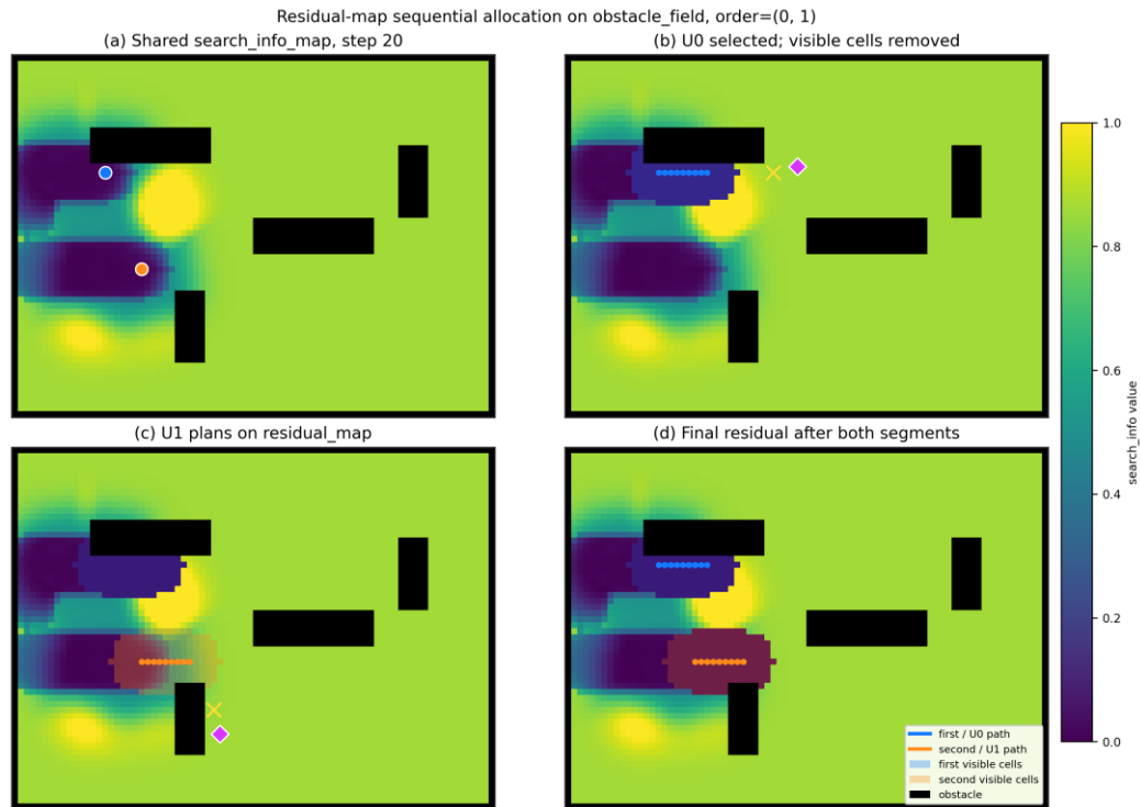
图 4-2 residual_map 顺序分配过程
